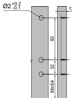
Крепление фасада
