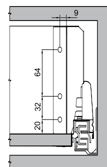
Задняя стенка
