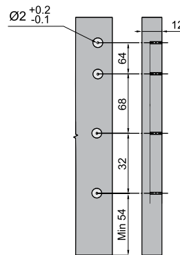
Крепление фасада
