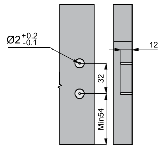
Крепление фасада
